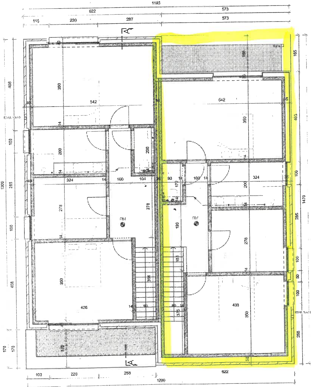
VERDIEPING 1/100
